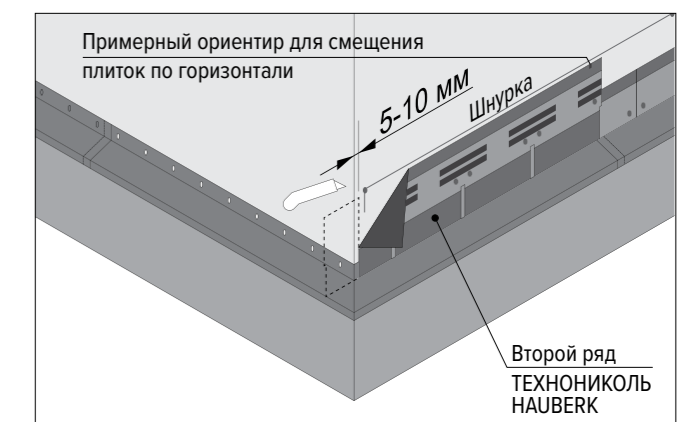
Рис. 8. Монтаж первого и последующих рядов фасадной плитки
