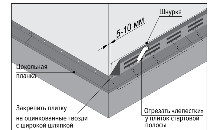
Рис. 7. Монтаж стартовой полосы фасадной плитки
