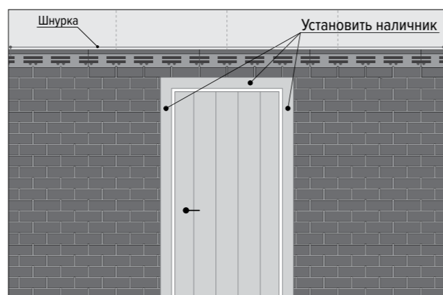
Рис. 12. Установка наличников
