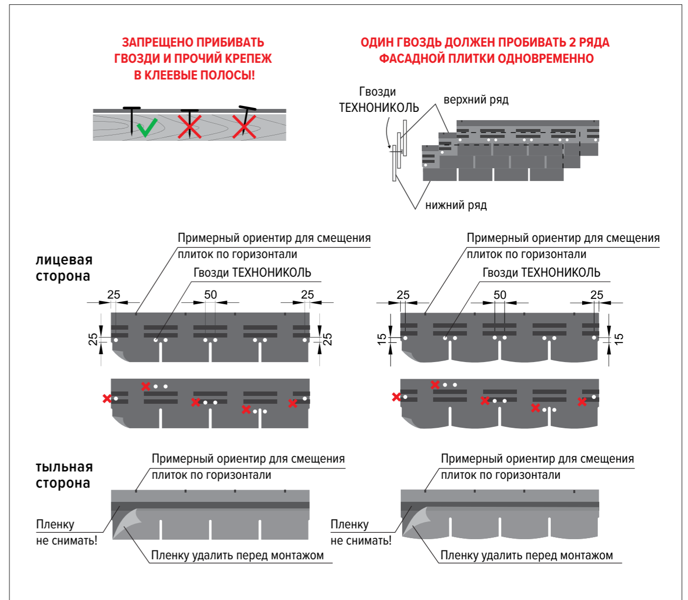
Рис. 2. Схема крепления фасадной плитки на 8 гвоздей
