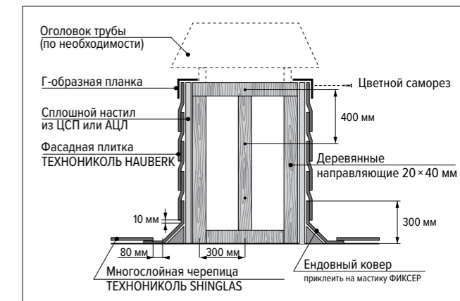
Рис. 26. Монтаж фасадной плитки на вентиляционную трубу
