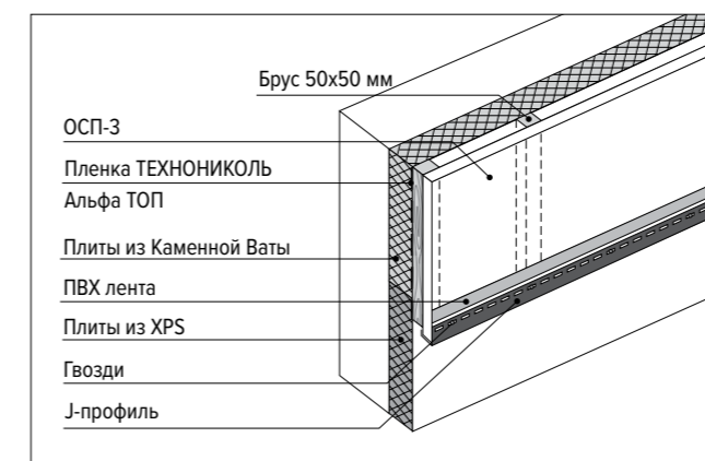
Рис. 6. Монтаж J-профиля
