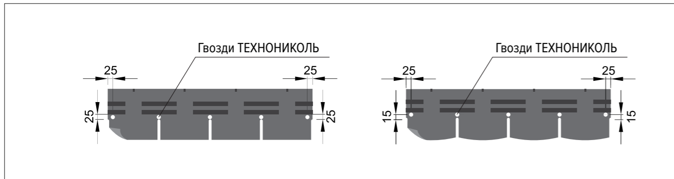
Рис. 3. Схема крепления фасадной плитки на 5 гвоздях
