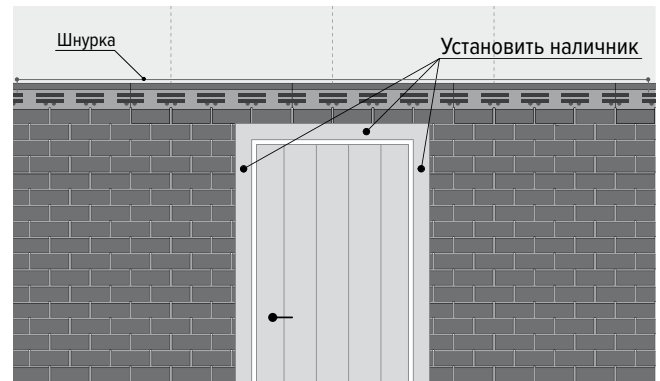
Рис. 16. Установка наличников
