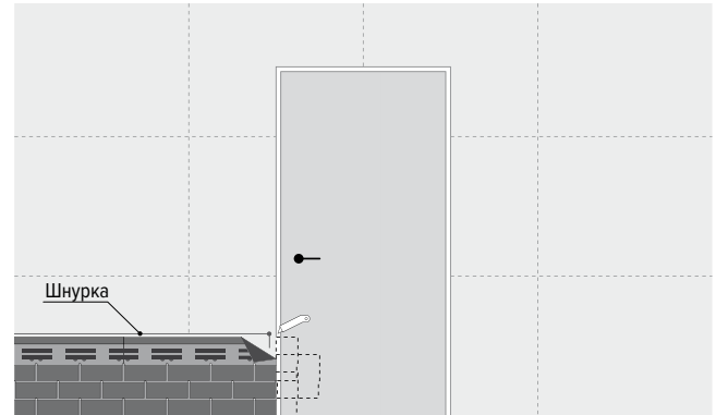
Рис. 15. Монтаж фасадной плитки вокруг дверных проемов
