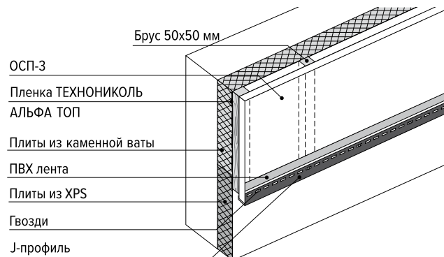
Рис. 7. Монтаж J-профиля
