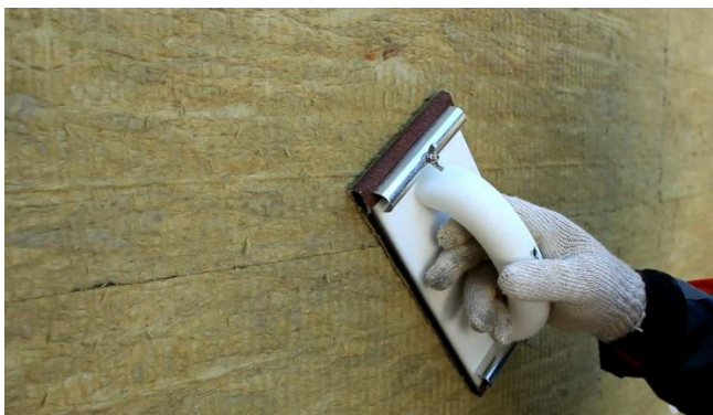
Рис. 12. Шлифовка стыков плит теплоизоляции наждачной бумагой
