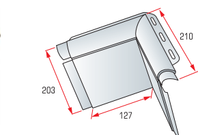
УГЛОВОЙ ЭЛЕМЕНТ ОТКОСА
