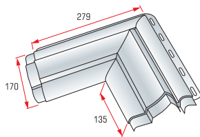
УГЛОВОЙ ЭЛЕМЕНТ НАЛИЧНИКА «КЛАССИК»
