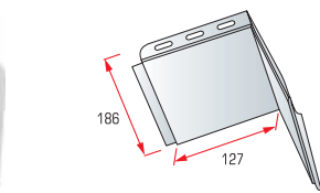
УГЛОВОЙ ДОБОРНЫЙ ЭЛЕМЕНТ К ОТКОСУ
