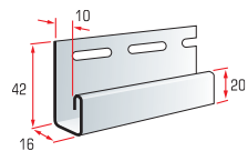
ПЛАНКА ОТДЕЛОЧНАЯ ДЛЯ ОТКОСОВ длина 3000 мм
